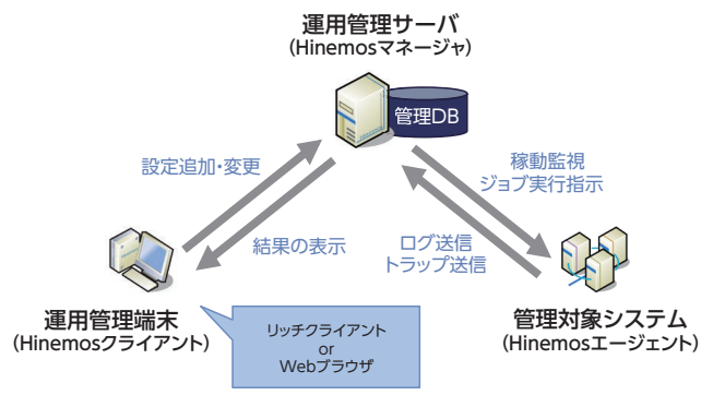
図1 Hinemosの構成
